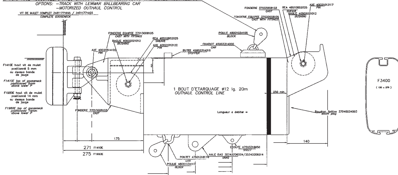
BOME F3400 AVEC MAT ENROULEUR F1410E-F1980E BOOM F3400 FOR FURLING MAST F1410E-F1980E
