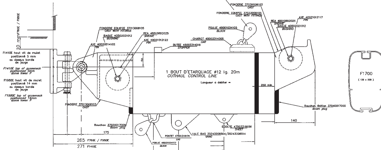
BOME F1700 AVEC MAT ENROULEUR F760E-F980E-F1410E BOOM F1700 FOR FURLING MAST F760E-F980E-F1410E
